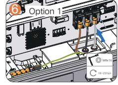
6-1 AC and equipotential bonding scheme 1
