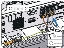
6-2 AC and equipotential bonding scheme 2
