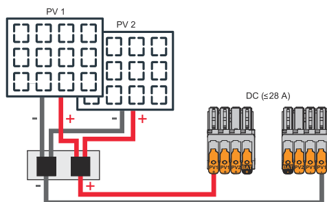
Stringhe di moduli solari combinate con corrente totale inferiore/uguale a 28 A ( I_{dcmax} ).
