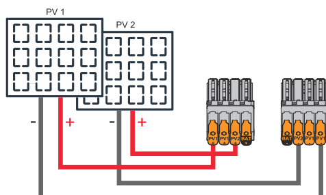
FV 1 inferiore o uguale a 40 A ( I_{SC\ PV1} ) FV 2 inferiore o uguale a 20 A ( I_{SC\ PV2} )
