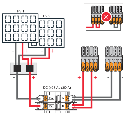
Stringhe di moduli solari combinate con corrente totale superiore a 28 A ( I_{dcmax} ).
